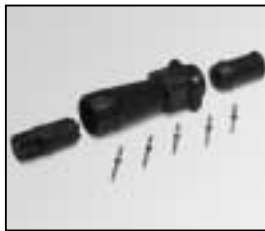
L4.76829.E Schaltbau connector (Female) 5 pins Schaltbaustecker (Buchsenkontakt) 5-polig
